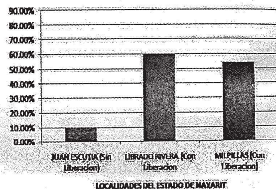
Figura 4. Comparación del porcentaje de parasitismo de ninfas de D. citri en tres localidades de los municipios de Compostela y San Pedro Lagunillas.
