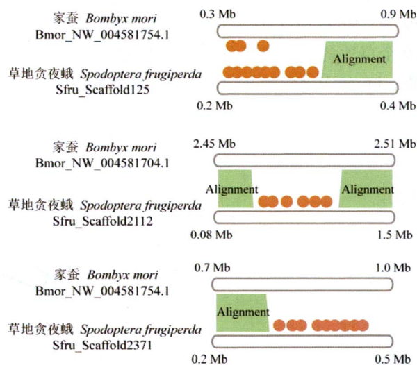
图 2 草地贪夜蛾与家蚕 P450 基因共线性分析 Fig. 2 Syteny analysis of the P450 genes of Spodoptera frugiperda (red) and Bombyx mori (blue)
