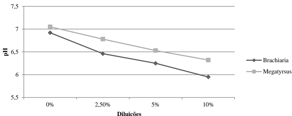
Figura 1. Valores médios do pH dos extratos de Brachiaria brizantha e Megatyrsus maximus em suas diferentes diluições (Cascavel (PR), 2017).
