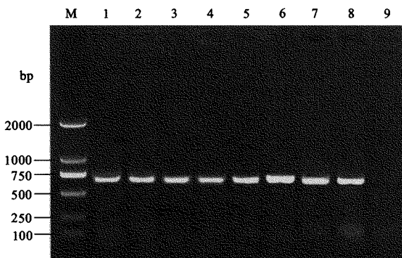
图 1 粉蚧 COI 基因通用型引物 PZTCOIF1/PZTCOIR1 对扶桑绵粉蚧及其他 7 种常见粉蚧的扩增结果电泳检测图
