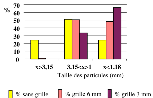
Figure 2. Profils granulométriques du maïs selon 3 types de broyage
